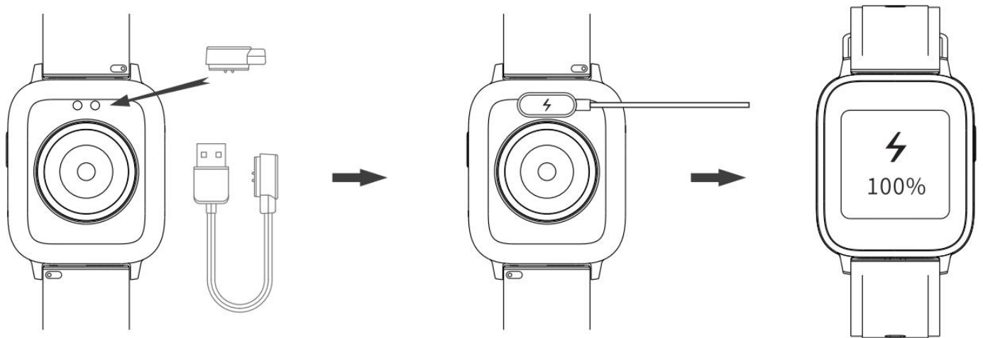
图 4-2 VDB1616 充电指导图/Charging Guide
